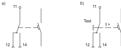
Рисунок 2 – Электрические схемы а) КС; б) КСВ / Picture 2 – Electric diagram a) KS; б) KSV
